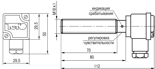
Габаритный чертеж.
